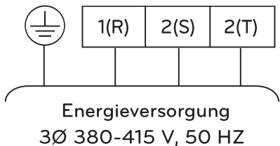
Klemmleiste 2 (in 3Ø Zusatzheizung)
