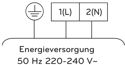
Klemmleiste 2 (in 1Ø Zusatzheizung)
