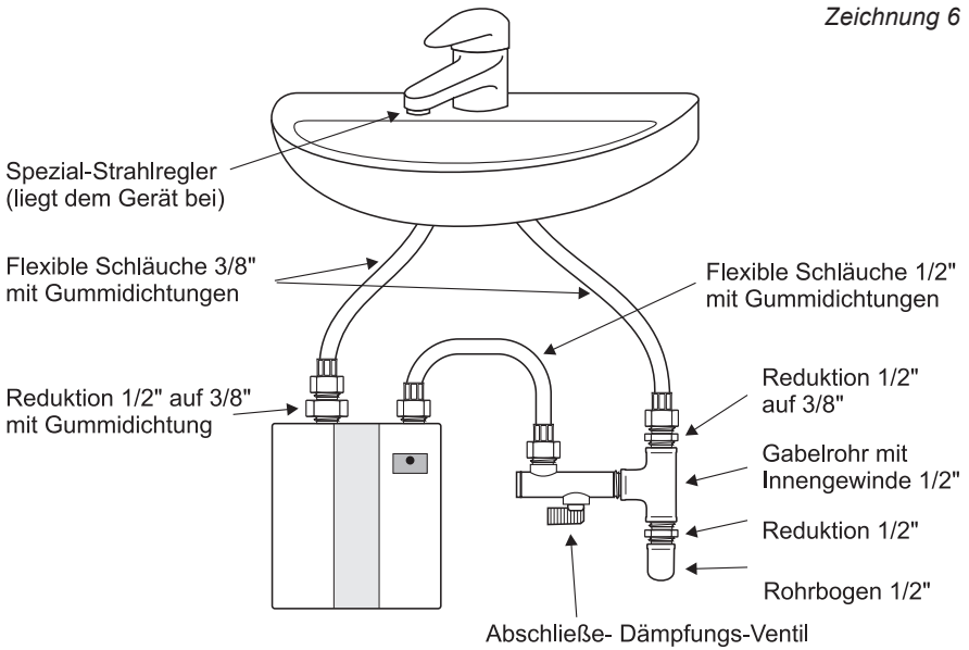
Anschließen des Durchflusswärmers an die Hahnatterie, ausgestattet mit den Schläuchen 3/8"
