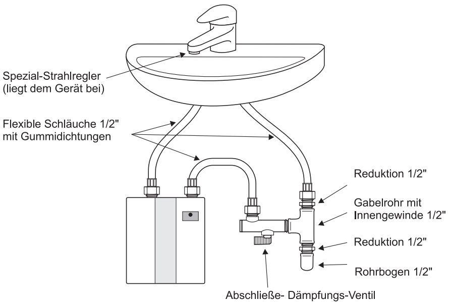
Anschließen des Durchflusswärmers an die Hahnatterie, ausgestattet mit den Schläuchen 1/2"
