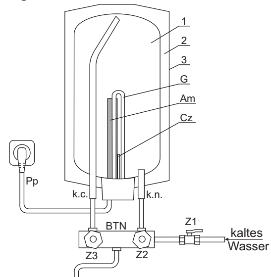
Abbildung 4. Montage des Tanks unter das Waschbecken in der Version nicht Druck.
