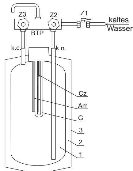
Abbildung 4. Montage des Tanks unter das Waschbecken in der Version nicht Druck.
